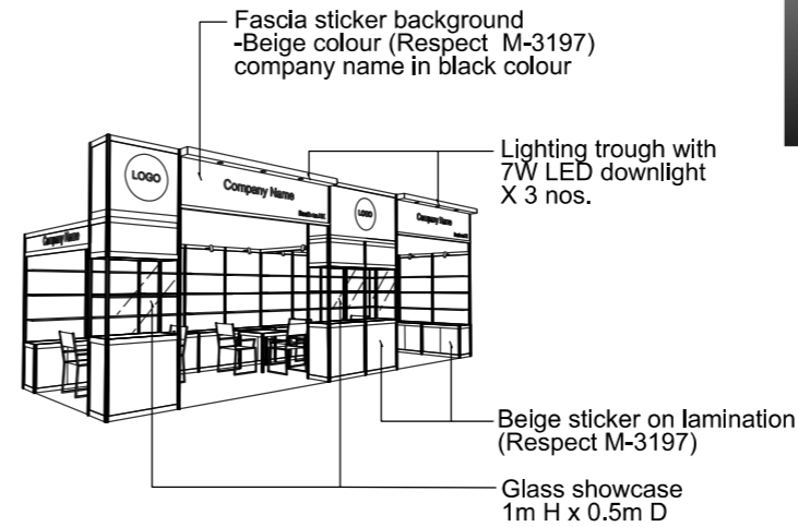
PERSPECTIVE N.T.S
