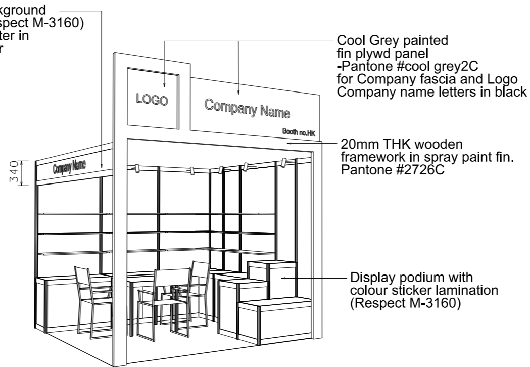
PERSPECTIVE N.T.S
