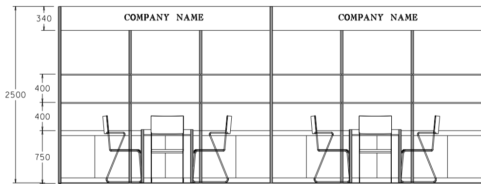
ELEVATION
