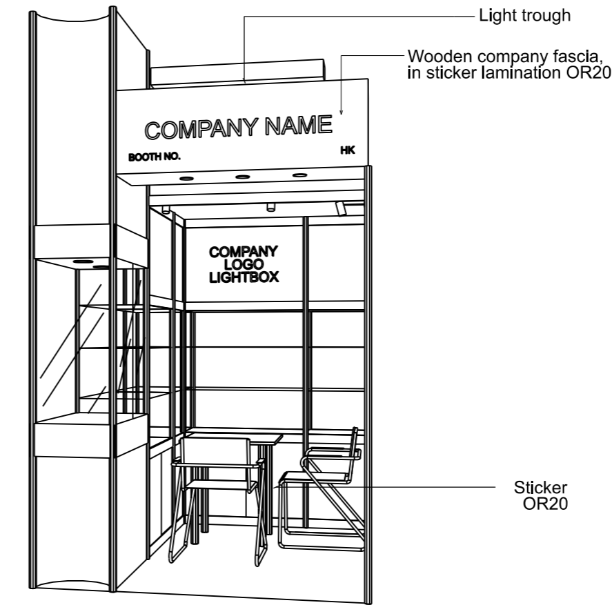
PERSPECTIVE N.T.S
